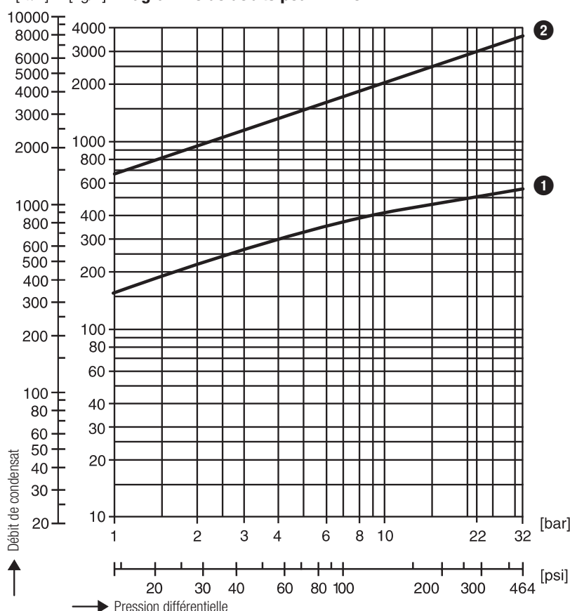
[lb/h] [kg/h] Diagramme de débits pour BK 46
